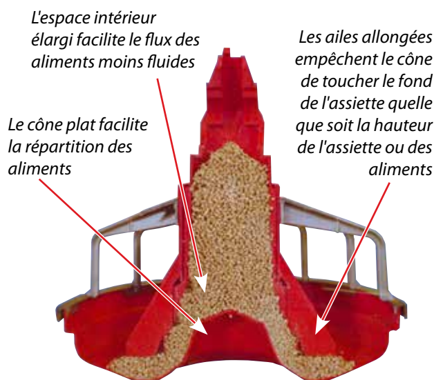
Modèle C2 PLUS Extensif ailette Nourrisseur de CHORE-TIME®
